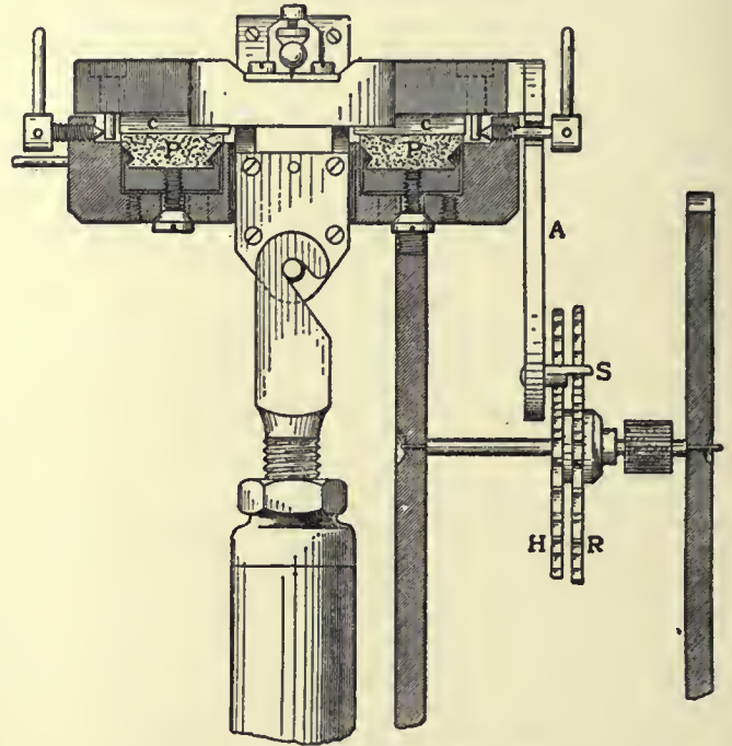
FIG. 11.—Riefler's Escapement.
